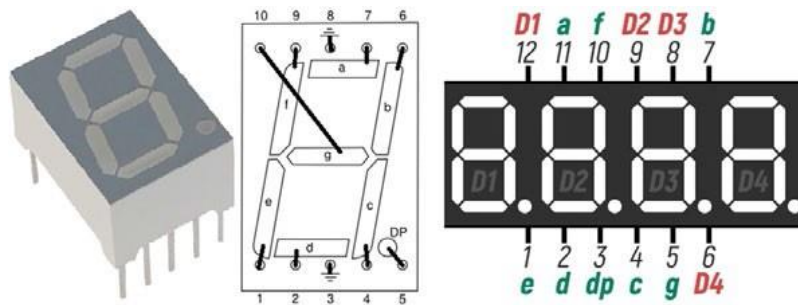
Рис. 13. Семисегментный индикатор и его распиновка
