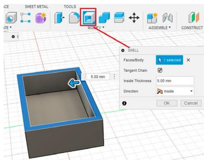
Рис. 13. Создание стенок корпуса с помощью SHELL
