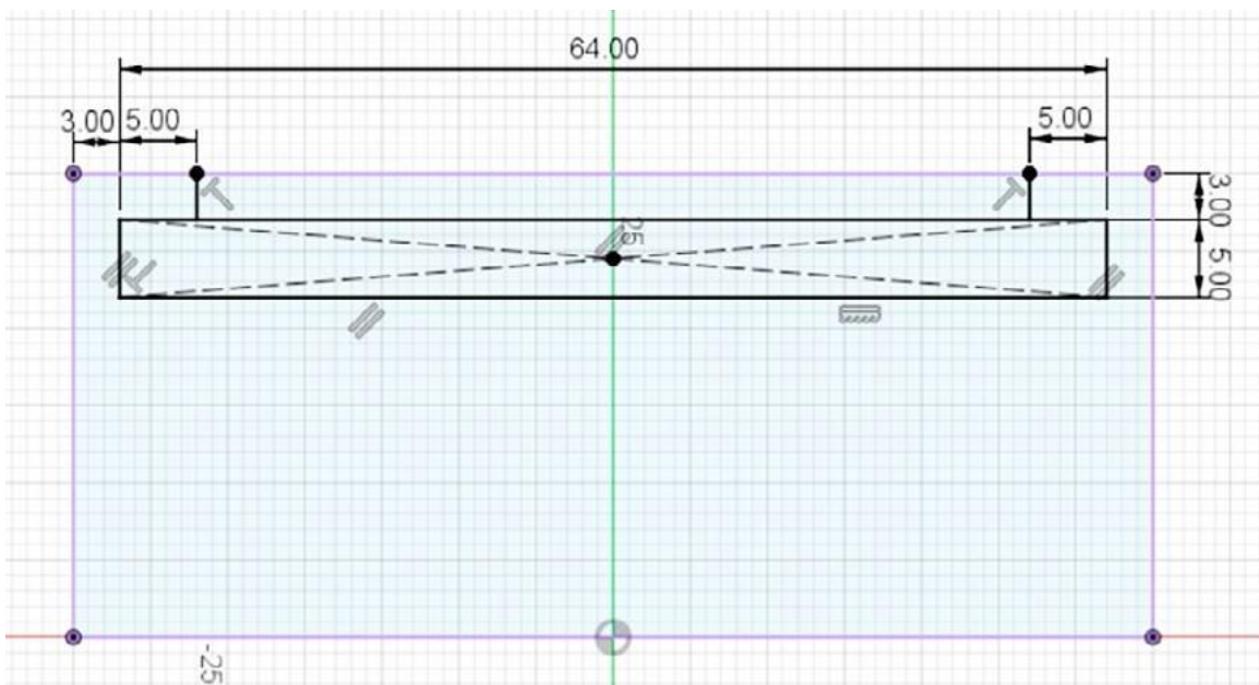
Рис. 15. Эскиз паза
